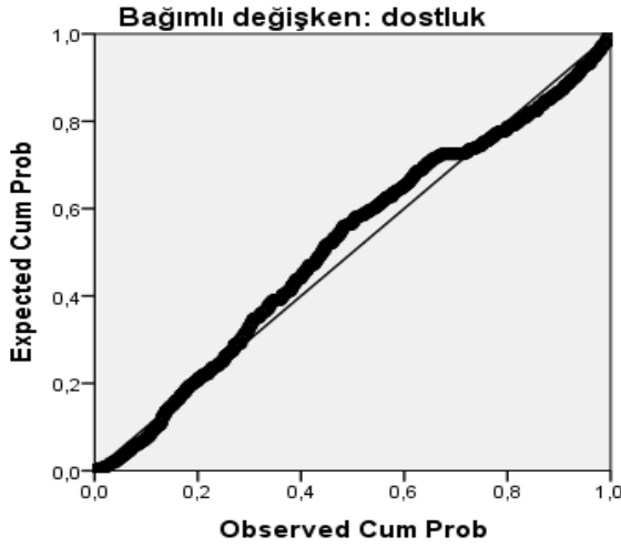
Şekil 1. Hataların Normal Dağılımı
